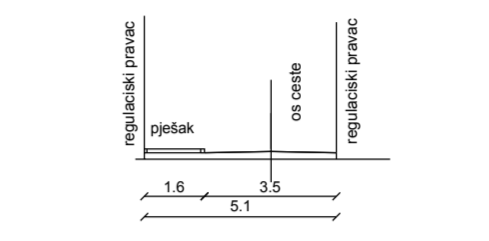
KARAKTERISTIČAN POPREČNI PRESJEK C - C M 1:200
