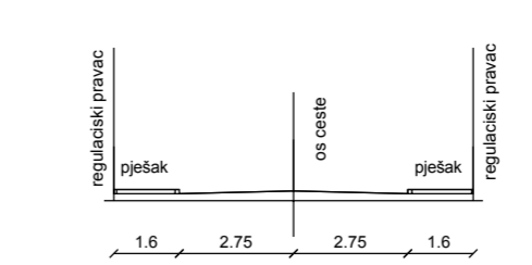
KARAKTERISTIČAN POPREČNI PRESJEK A - A M 1:200
