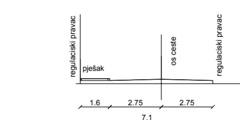
KARAKTERISTIČAN POPREČNI PRESJEK B - B M 1:200
